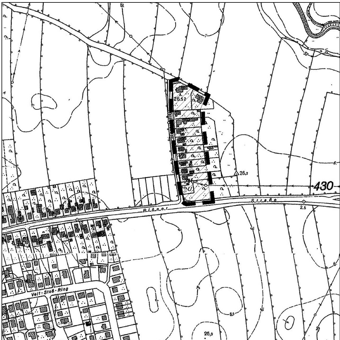
Übersichtsplan M 1 : 5.000
